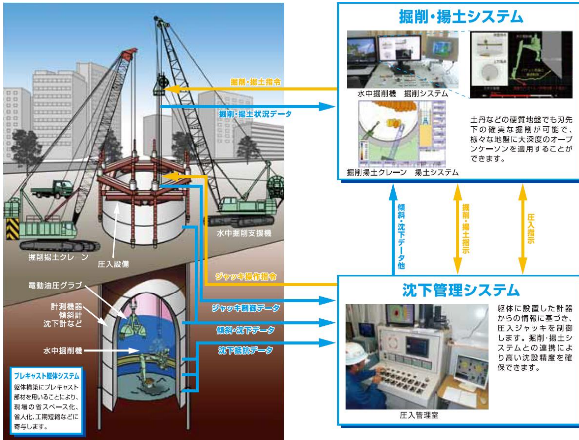
システム全体図
