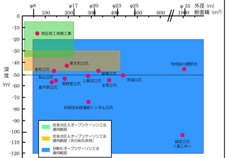
各工法の適用範囲とSOCS施工実績
