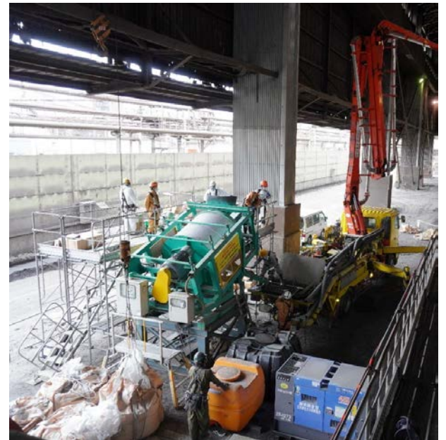
図-8 ポリマーコンクリート現場打設状況
