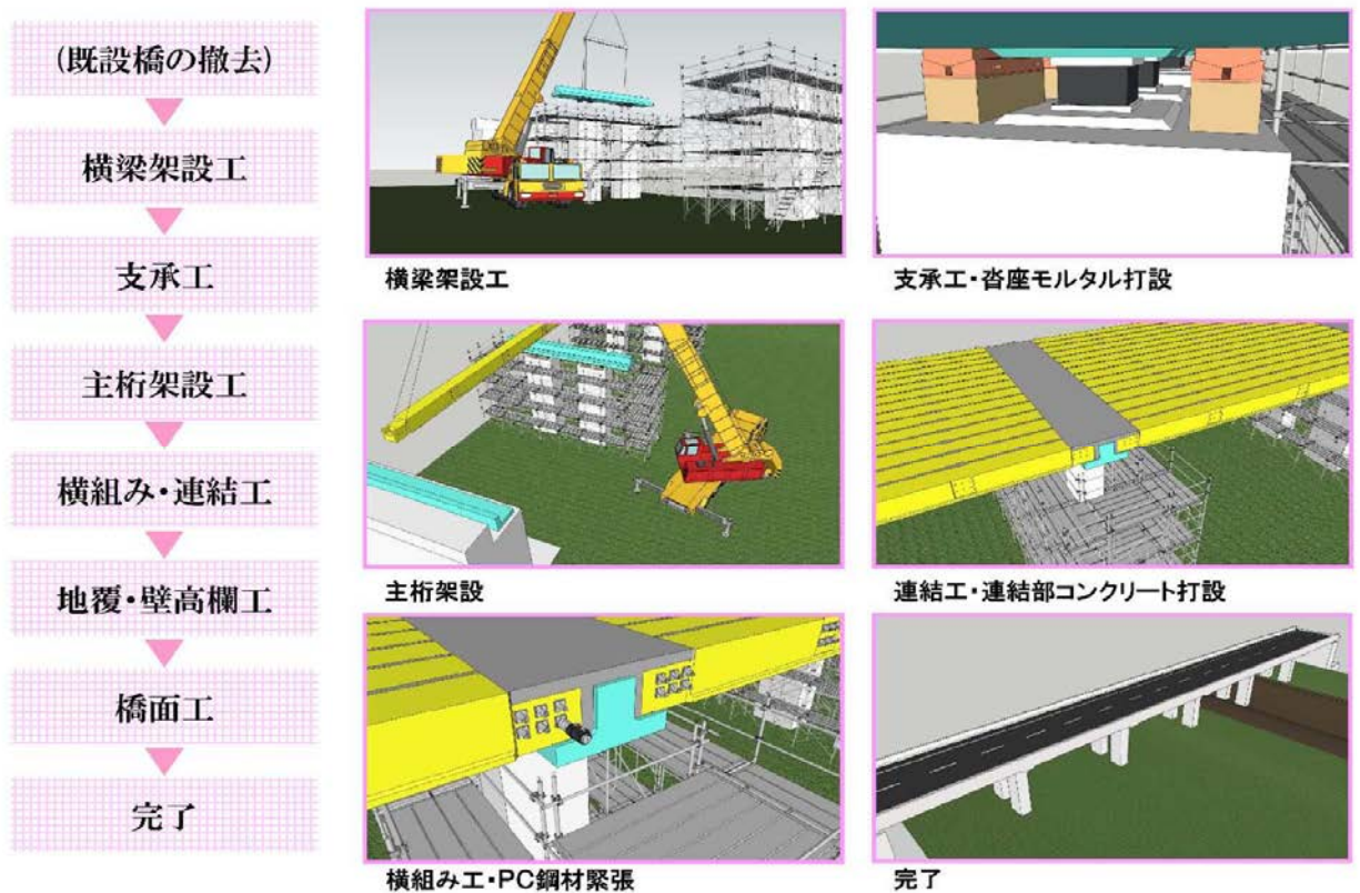
図-2 SCBR工法の施工ステップ
