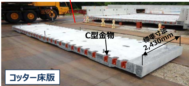
写真-1 橋梁用「コッター床版工法」の概要
