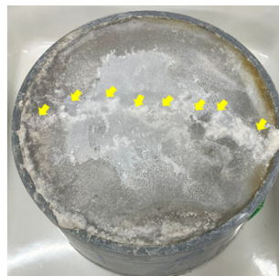
ひび割れ幅：0.30mm 測定材齢5週で止水
