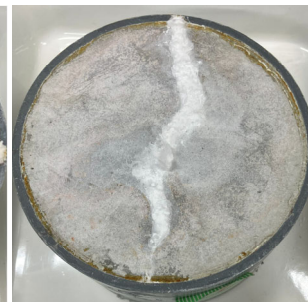
ひび割れ幅：0.28mm 測定材齢6週で止水
