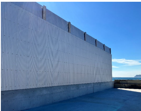
BiSCoを打設した防潮壁
