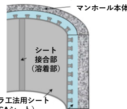
スラスラ工法の概念図
