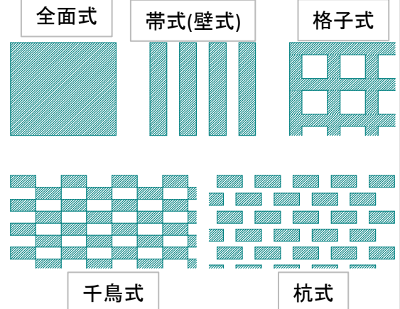
図-2 改良形式図(例)
