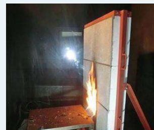
【JSP】 火災時想定実験
