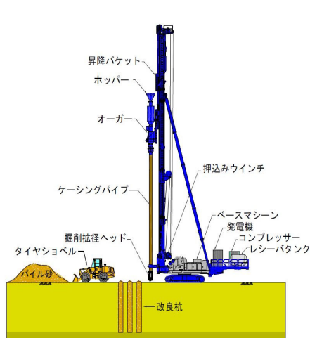
施工概要図 Construction outline
