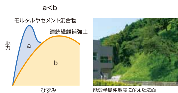
応力-ひずみ曲線
