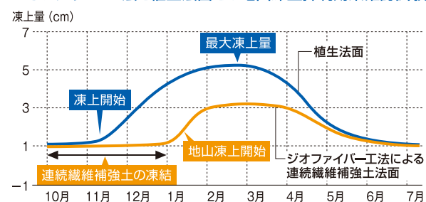
ジオファイバー工法と植生法面との地山凍上抑制効果確認試験
