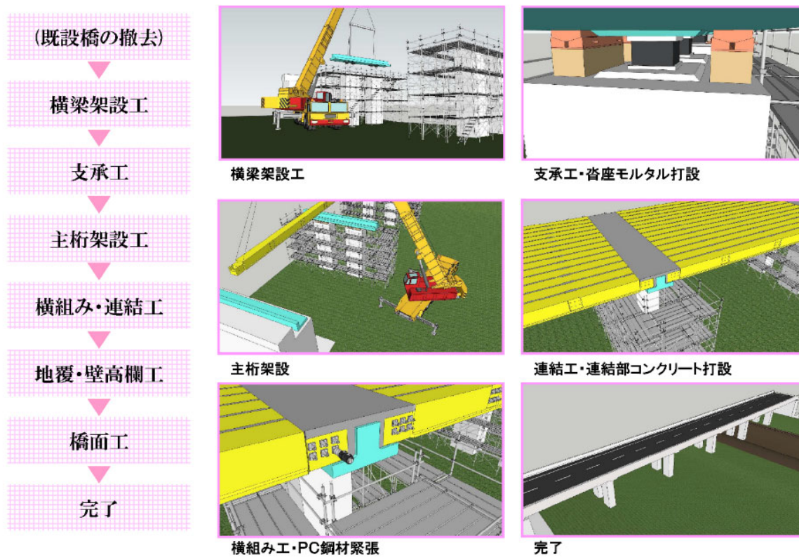
図－2 SCBR工法の施工ステップ
