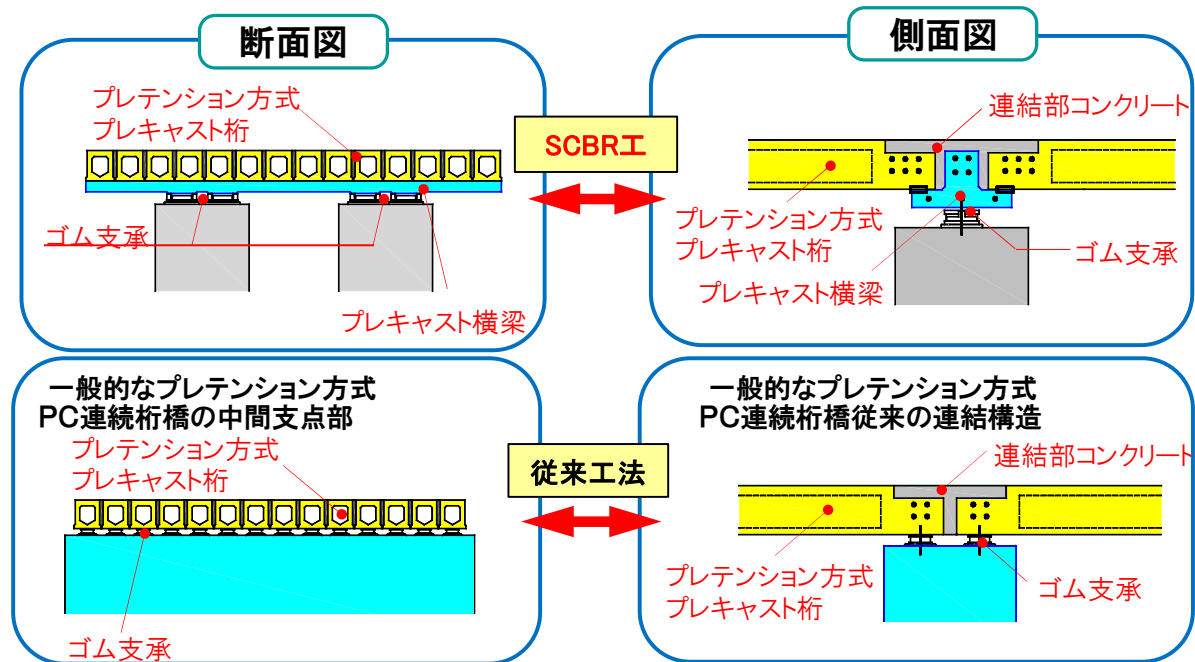
図－1 プレテンション方式PC連続桁橋の従来工法とSCBR工法の違い
